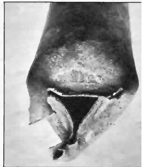
Für den bei Kilometerstand 7 585 auftretenden Leistungsverlust war das Auspuffrohr verantwortlich, das in den zweiten Schalldämpfer mündete. Es hatte sich aufgrund hoher Temperaturen stark verformt und behinderte dadurch die Abgase auf ihrem Weg ins Freie.
