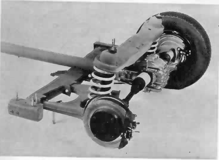
Das sorgfältig abgestimmte Fahrwerk mit Federbeinen vorn (links oben) und Schräglenker-Hinterachse (darunter) sorgt für überdurchschnittlichen Komfort und sichere Fahreigenschaften. Die wichtigsten Aggregate des Einspritzmotors (oben) sind gut zugänglich.
