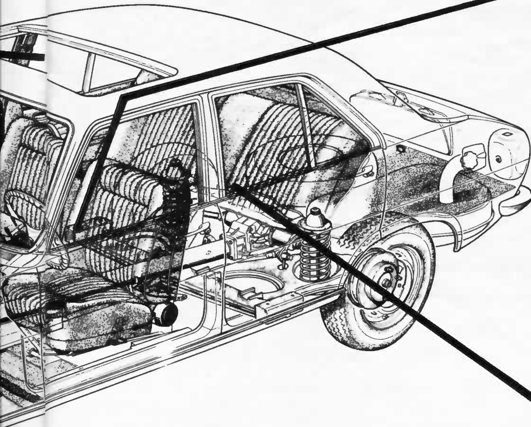
Für den bei Kilometerstand 7 585 auftretenden Leistungsverlust war das Auspuffrohr verantwortlich, das in den zweiten Schalldämpfer mündete. Es hatte sich aufgrund hoher Temperaturen stark verformt und behinderte dadurch die Abgase auf ihrem Weg ins Freie.
