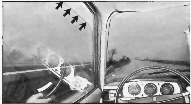
Die vorderen Seitenscheiben ließen sich bei hohem Tempo zwar öffnen, aber nicht mehr ganz schließen, weil sie vom Windsog nach außen gezogen wurden.
